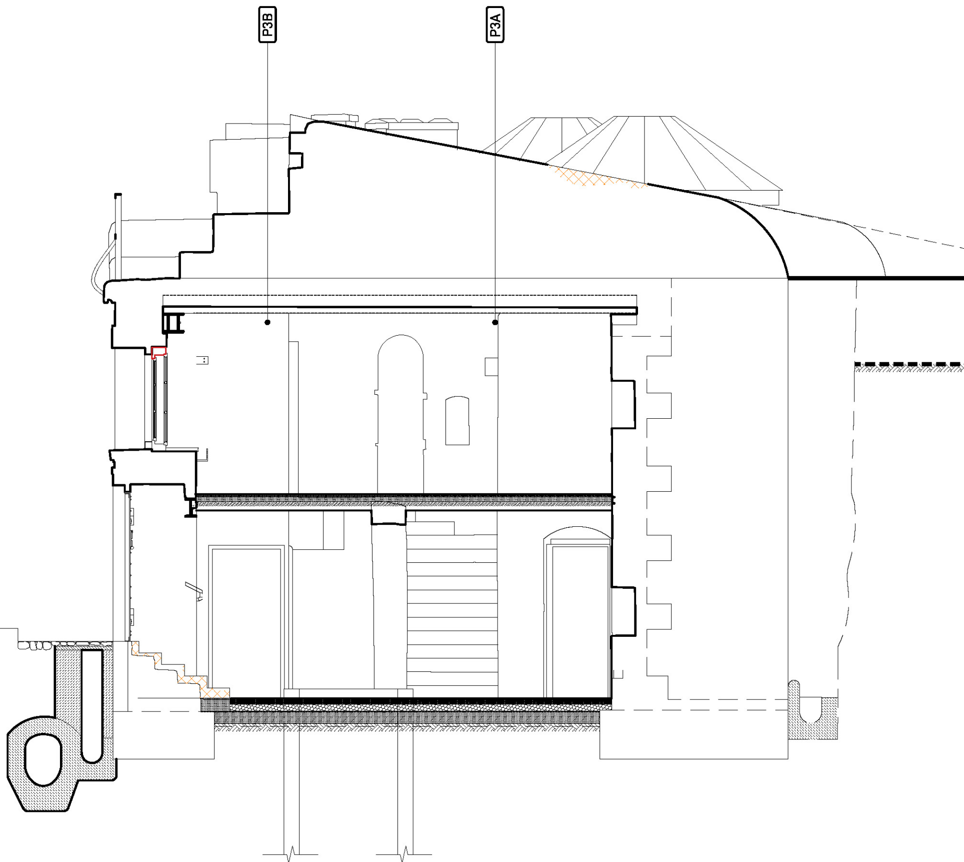
przekrój b-b
