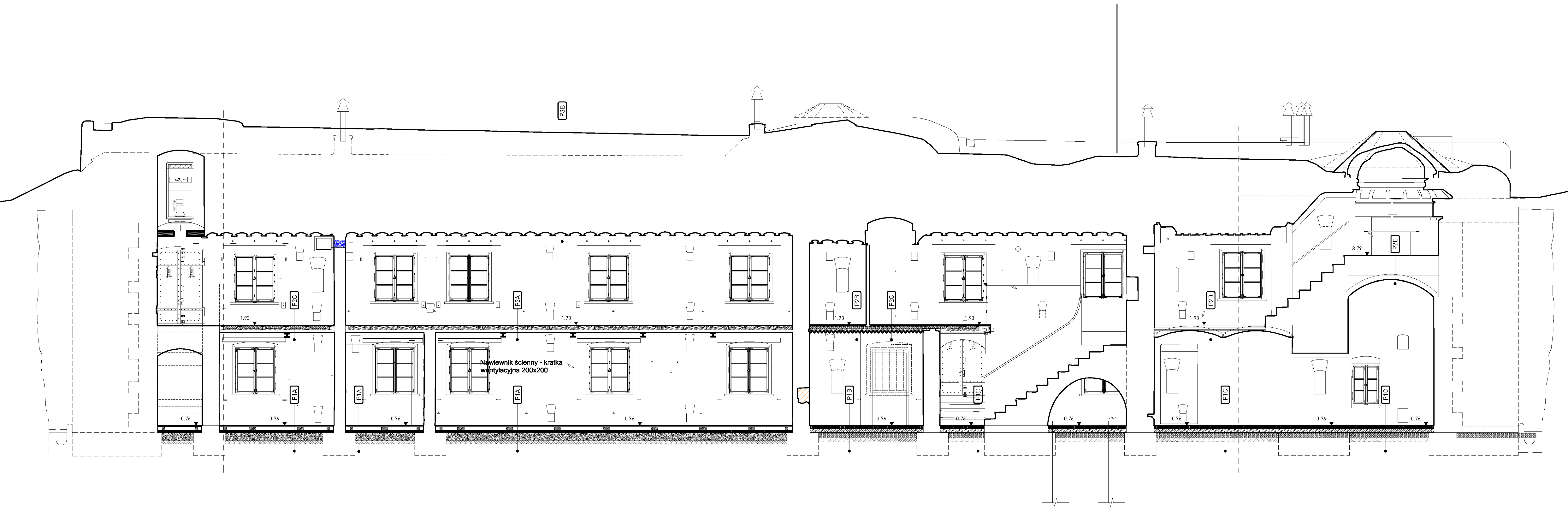
przekrój a-a
